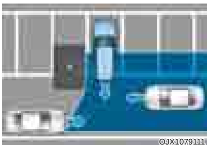
[A]: 构造物
