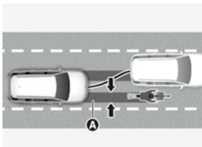
[A] 避撞转向辅助功能的操作空间
