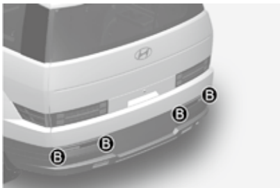
[A] 后视广角摄像头 [B] 后超声波传感器
