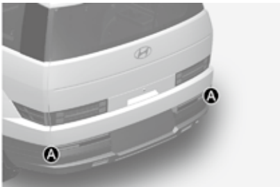
[A] 后侧面雷达传感器 检测传感器的具体位置请见上图。
