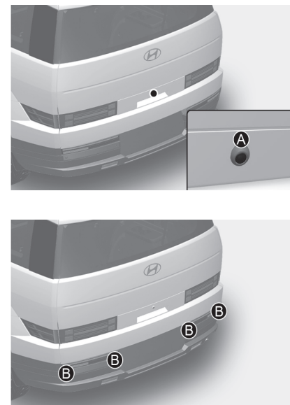
[A] 后视广角摄像头 [B] 后超声波传感器
