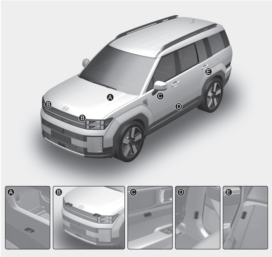
[A] 辅助保护系统控制模块 (SRSCM) / 侧翻传感器 (如有配备) [B] 正面碰撞传感器 [C] 侧面碰撞传感器 (压力式): 前车门 (如有配备) [D] 侧面碰撞传感器 (加速度式): B- 立柱 (如有配备) [E] 侧面碰撞传感器 (加速度式): C- 立柱 (如有配备)
