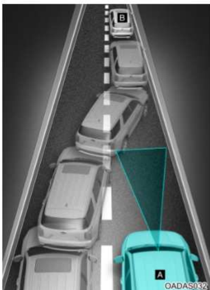
[A]: 您的车辆, [B]: 车道变更车辆
